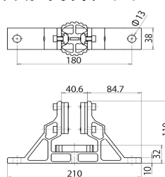
アンカーブラケット4040
