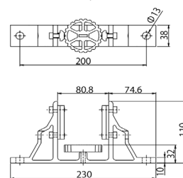
アンカーブラケット4080
