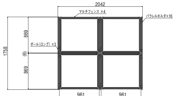
マルチフェンス+ボール(ロング) + 連結(パラレルホルダー)
