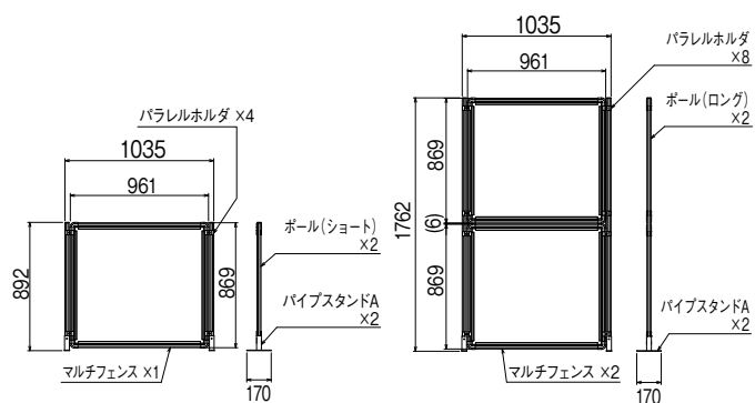
マルチフェンス+ボール(ショート/ロング) + パイプスタンド
