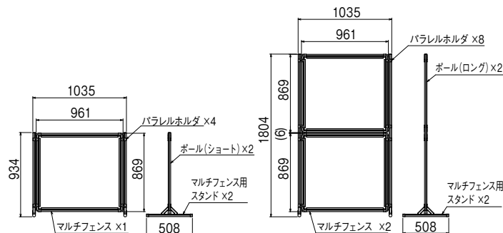
マルチフェンス (連結イメージ)
