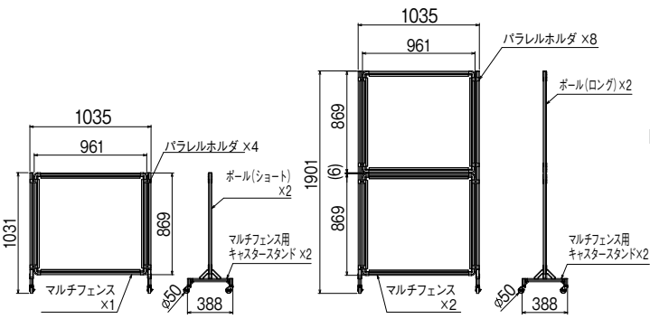
マルチフェンス+ボール(ショート/ロング) + キャスタースタンド
