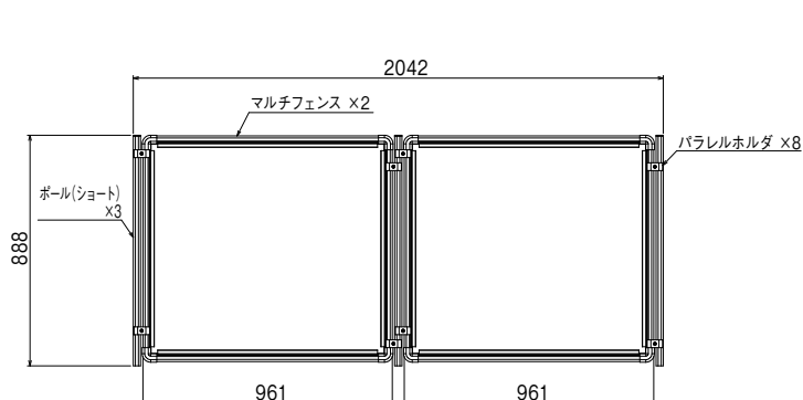
マルチフェンス+ボール(ショート) + 連結(パラレルホルダー)
