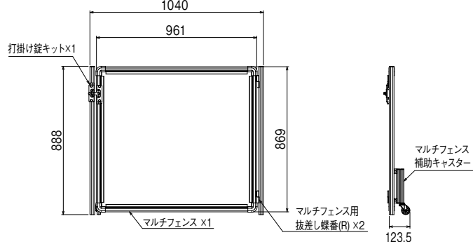
マルチフェンス+ボール(ショート) + 蝶番 + 内掛け錠又は取手
