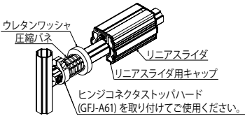
■ 使用例 リニアスライダ
