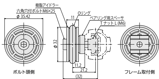
樹脂アイドラー Oリング取付キット (GFK-965)
