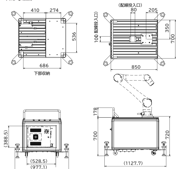
外形寸法図
