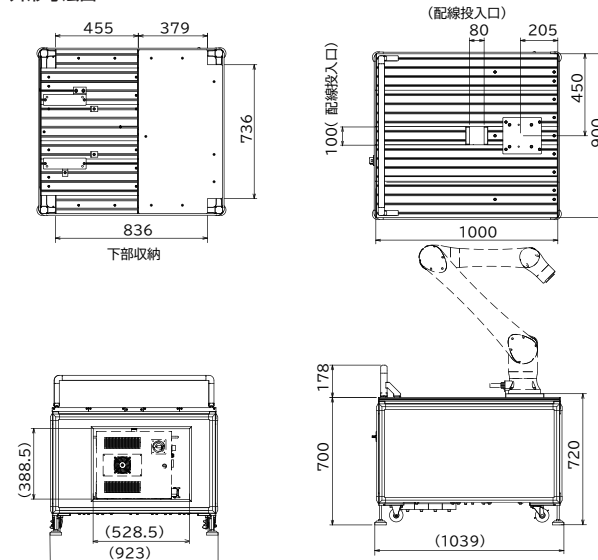
外形寸法図
