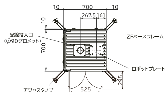
外形寸法図
