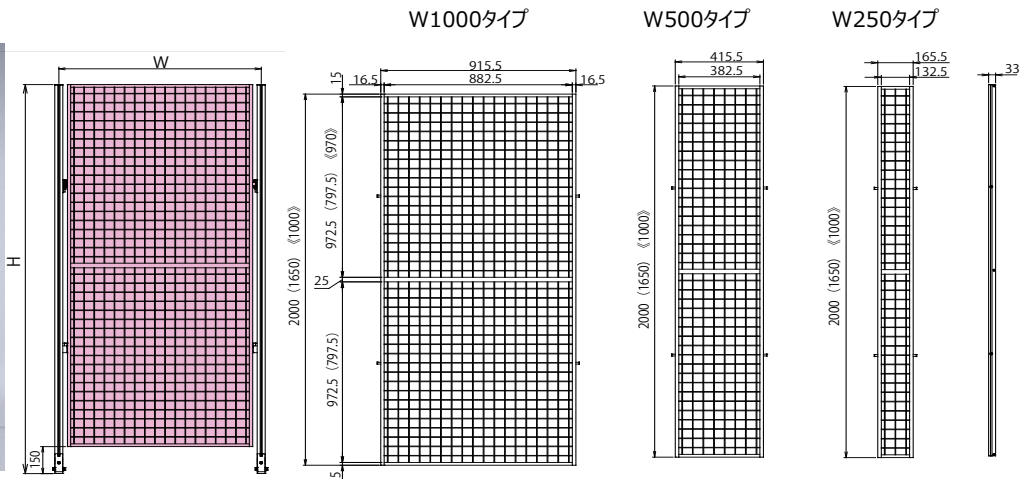
■寸法図
