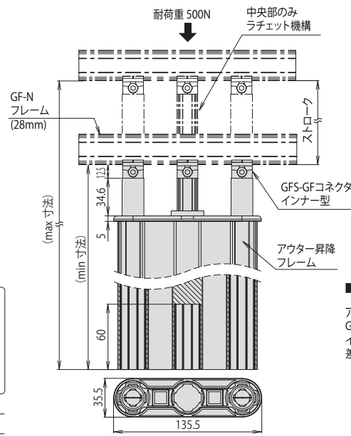
アウター昇降フレーム寸法 (キャップ含まず)
