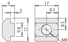
アルミTナットL (M8)
