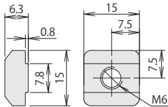
アルミTナットS (M6)
