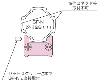
CYL-G31S 取付図
