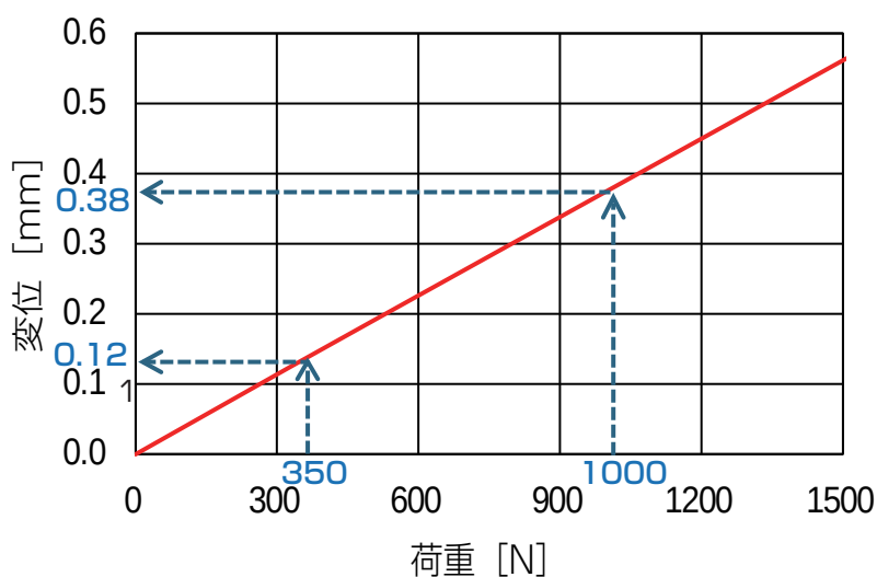
図 荷重-変位グラフ
