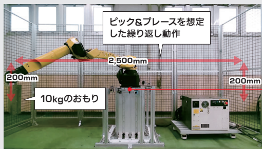
耐久試験の様子
