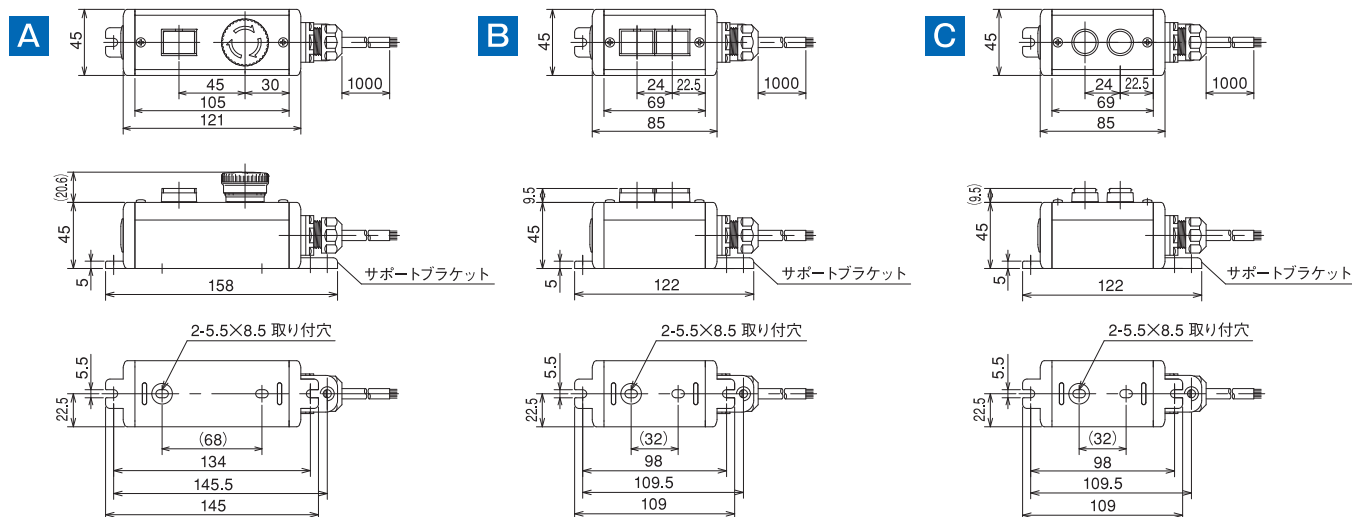
φ16スイッチ(頭部φ30)用 非常停止ガードS
