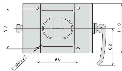
チルトジョイントL ボックス背面取り付け
