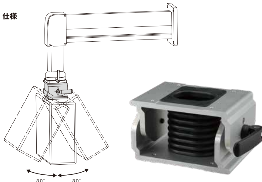
モニターアーム4LL・3LL・2LL・4L・3L・2L+チルトジョイントL モニターアーム1L+チルトジョイントL
