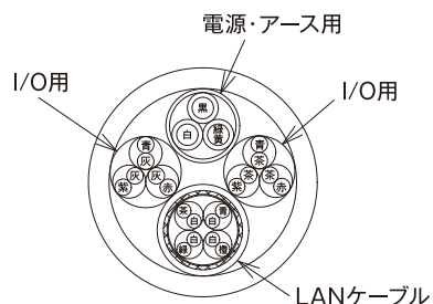
複合ケーブル(アース線+I/O6芯+電源+LAN)
