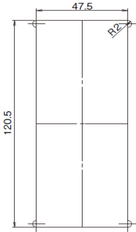
パネル穴あけ寸法
