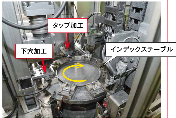
加工機の内部。ワークはインデックステーブルで順番に加工工程へ送られる。
