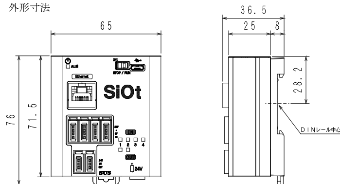
外形寸法
