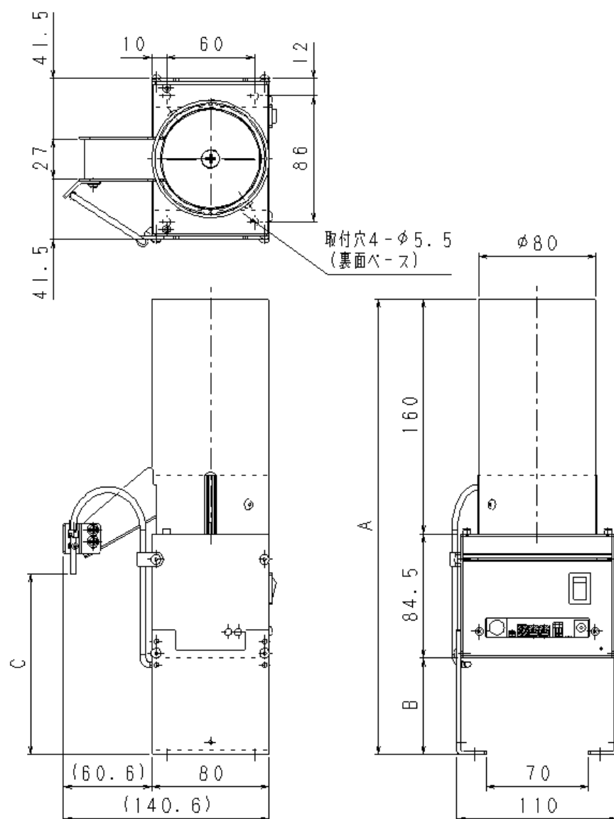
単体寸法図
