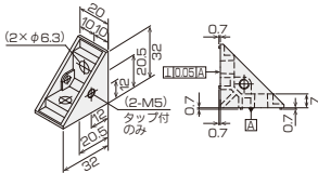
CブラケットS
