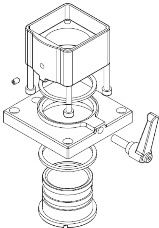
ターンマウントM分解図
