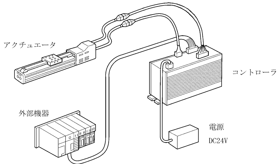
本図はエンコーダ付きアクチュエータを接続した図
