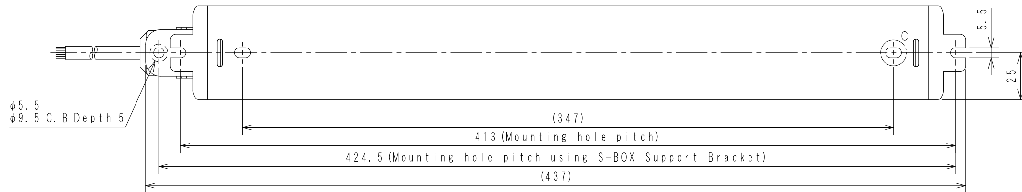
A-A View
