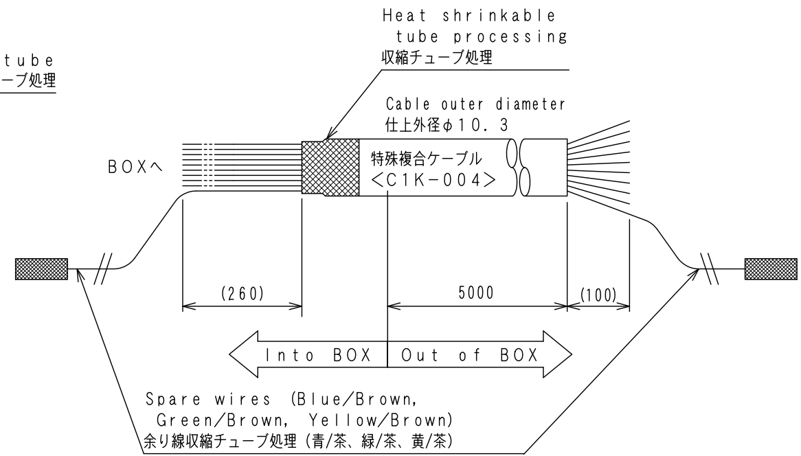
ケーブル処理詳細 Detail of cable
