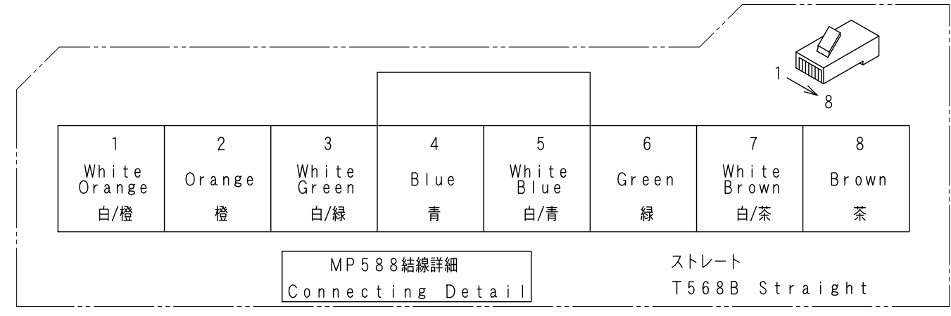
ケーブル処理詳細 Detail of cable
