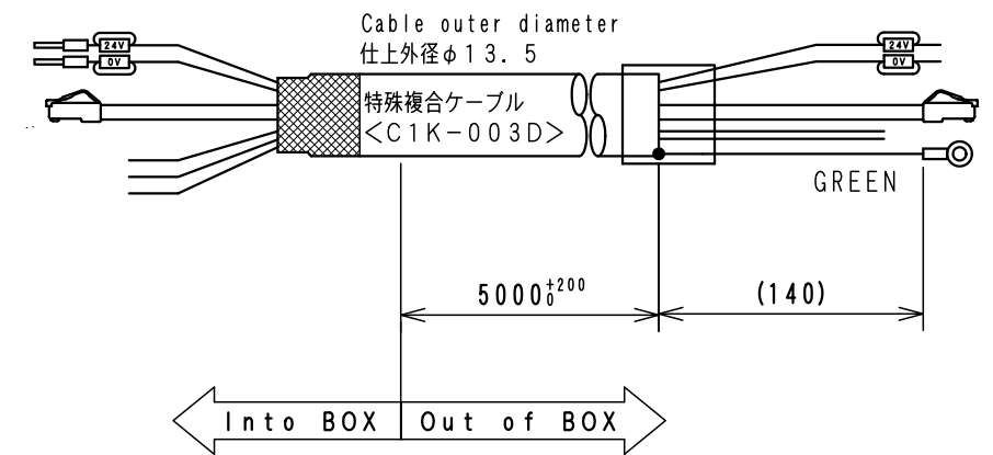
ケーブル処理詳細 Detail of cable
