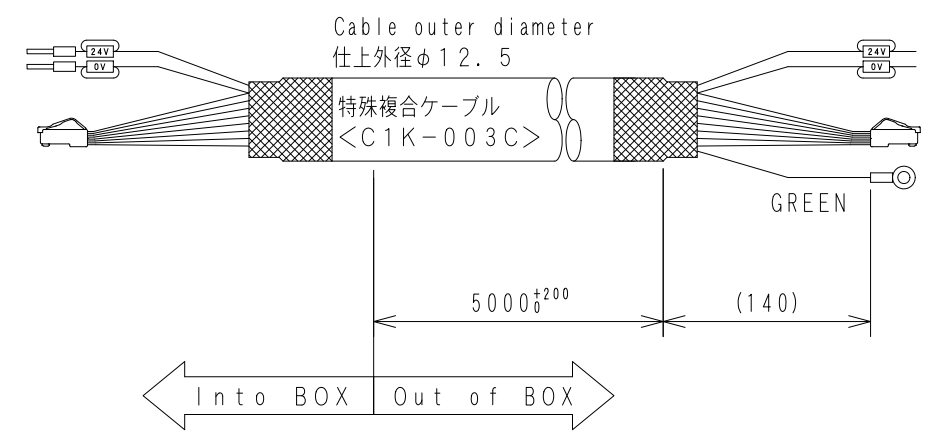
ケーブル処理詳細 Detail of cable
