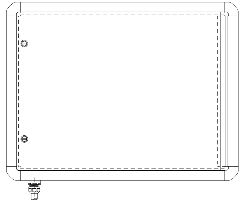
A-A View
