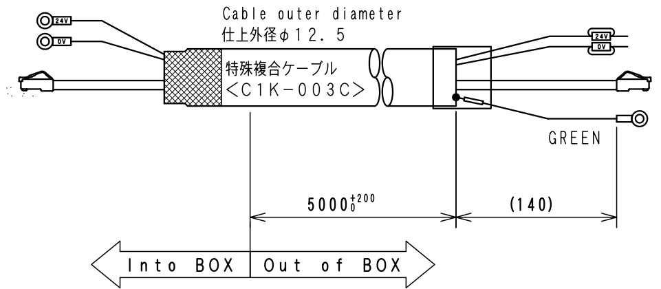
ケーブル処理詳細 Detail of cable
