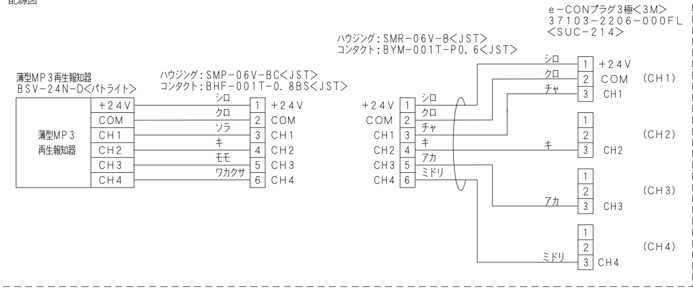
配線図
