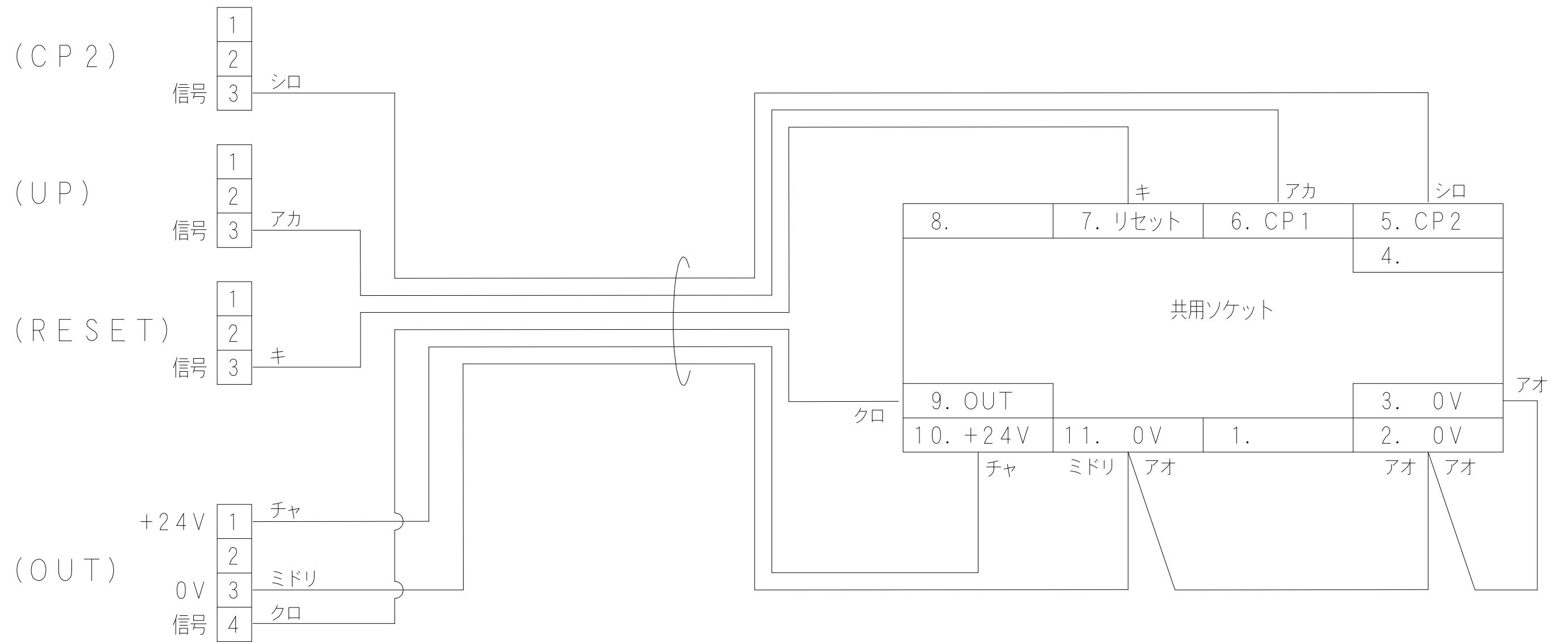
共用ソケット配線図
