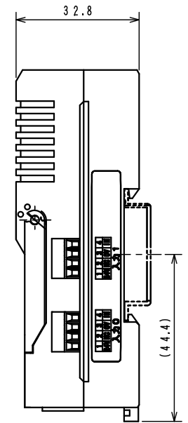
れんら君側面図
